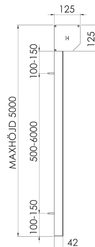
Byggmått gavel
