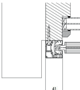
Byggmått nedfäld
