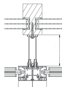
Byggmått gavel
