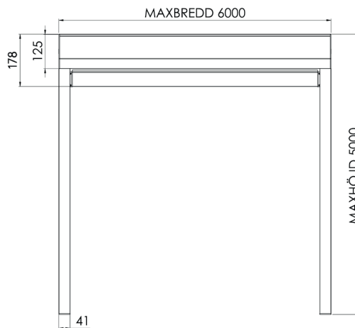
Byggmått uppfäld
