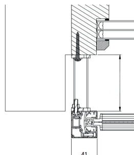
Byggmått uppfäld
