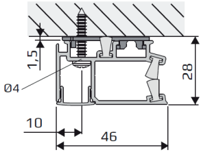
Takmontage med skruv
