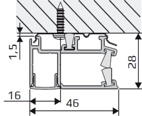
Takmontage med clips
