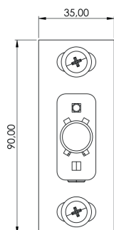
Byggmått distansfäste
