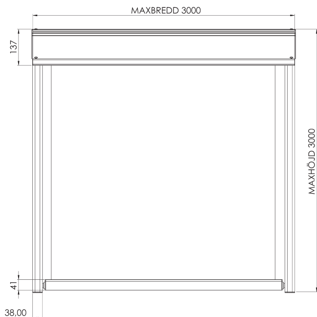
Byggmått nedfälld
