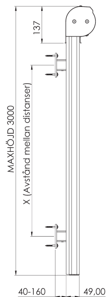
Byggmått gavel
