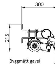
Byggmått gavel
