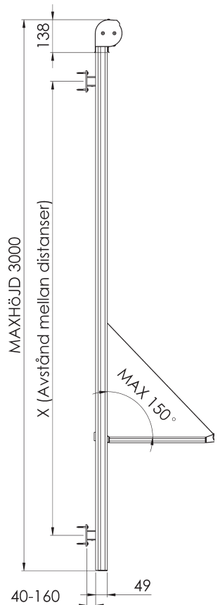
Byggmått sidovy utfäld
