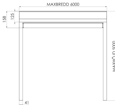
Byggmått uppfäld
