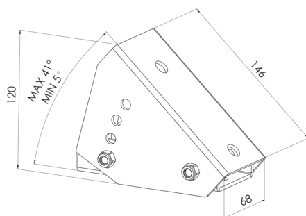
Ställbar takstolskonsol
