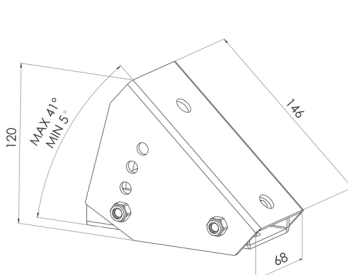
Ställbar takstolskonsol
