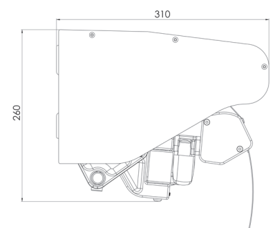
Byggmått gavel med tak
