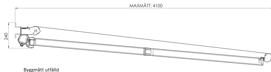
Byggmått utfälld
