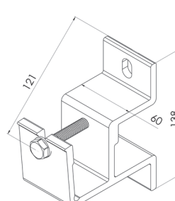
Kombikonsol
