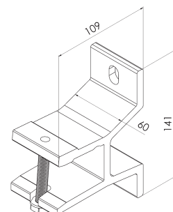
Väggkonsol
