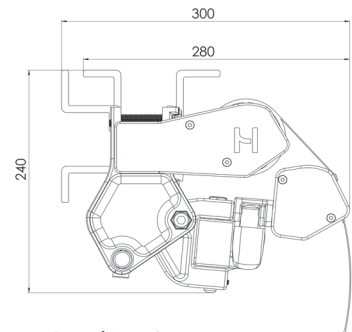
Byggmått gavel
