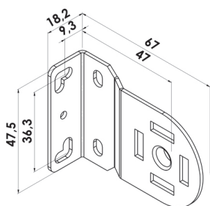
Gavelbeslag för tak, vägg och nisch
