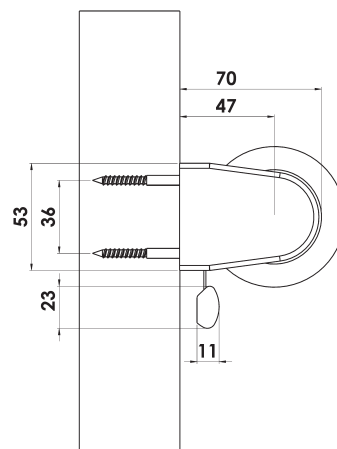
Tillval - synlig bottenlist
