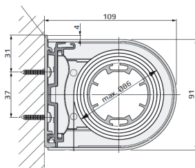
Modell 20 = Monteringsskena
