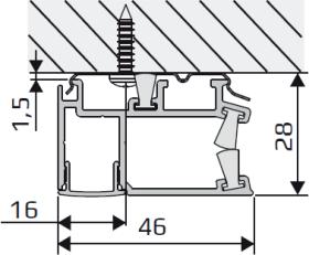
Takmontage med clips
