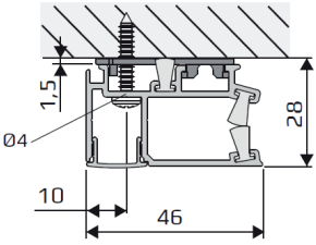
Takmontage med skruv
