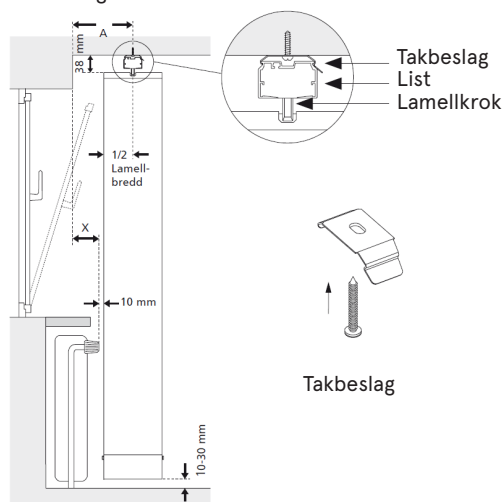
Montering i tak
